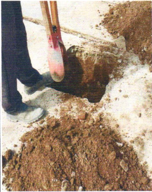
ESCAVAÇÃO MANUAL PARA SAPATA ISOLADA
