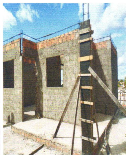
MONTAGEM E CONCRETAGEM DE PILARES
