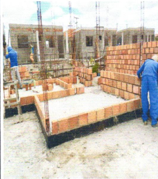
LEVANTE DE ALVENARIA
